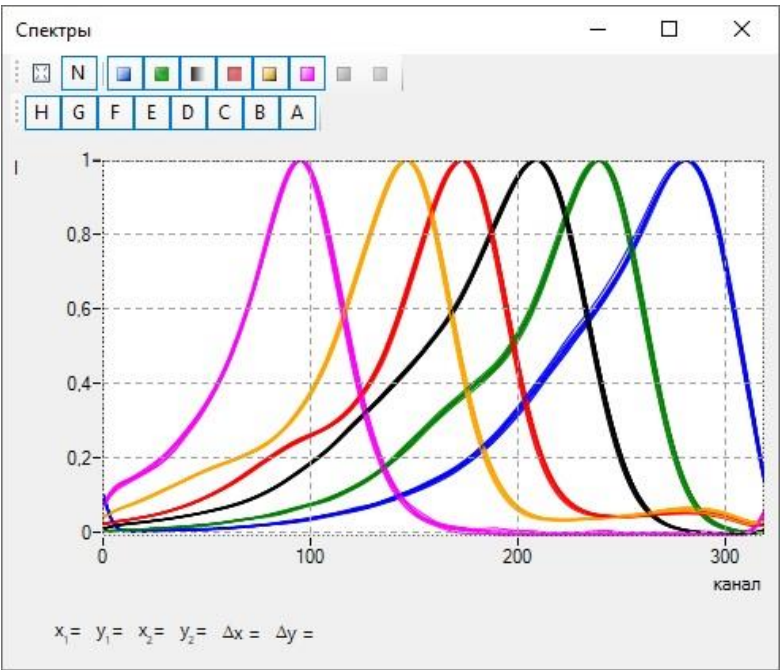
DS-36. Спектры набора красок:
