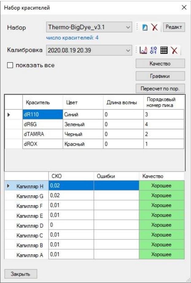
BigDye v3.1. Вид окна при успешно прошедшей калибровке набора:
