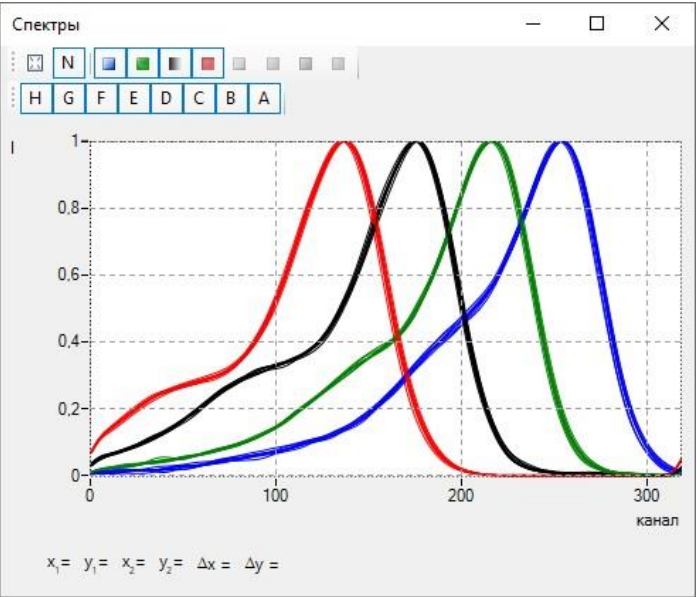
BigDye v1.1. Спектры красок набора:
