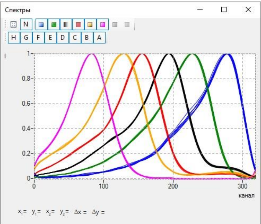
СК-6. Спектры красок набора:
